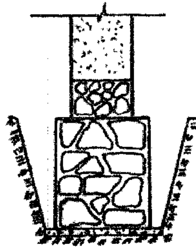
أ- أساس برذمات الأحجار
