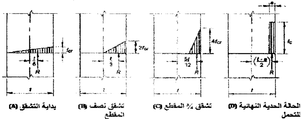
الشكل 29. توزيع إجهادات المضاطعة لمختلف حالات التشوه
