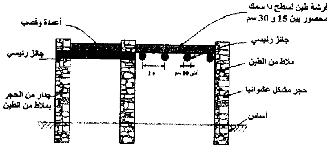
الشكل.11. رفع لبناية تقليدية بالحجر
