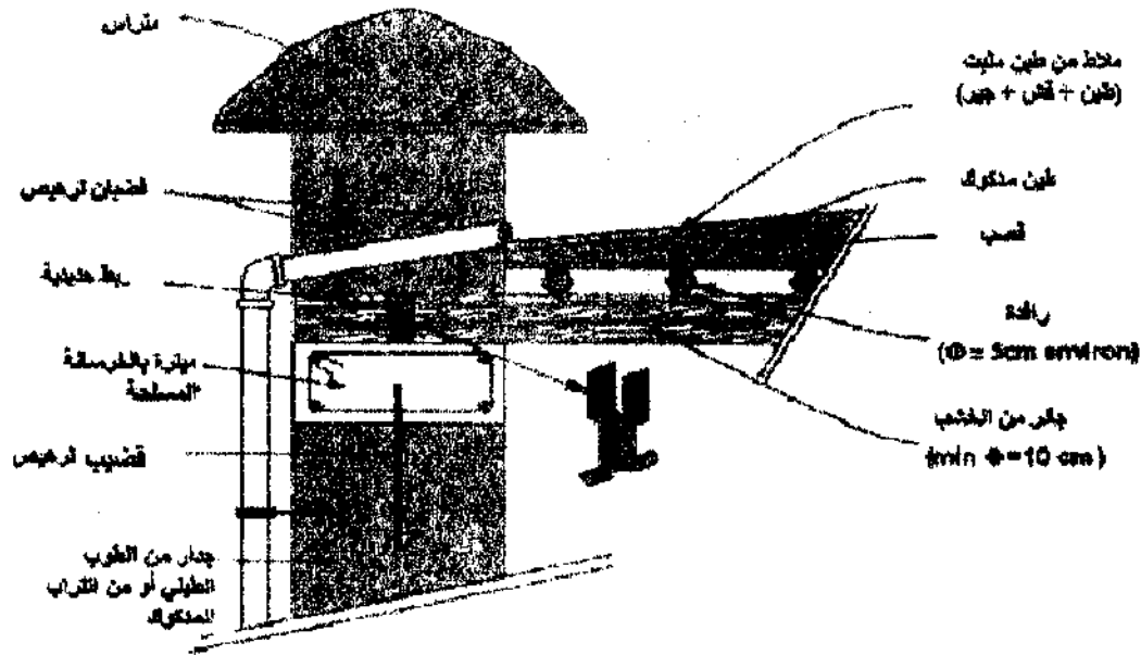
الشكل 38. ميترة أفقية بالخرسانة المسلحة، سقف تقليدي وربط جدار-ميترة أرضية-ميترة
