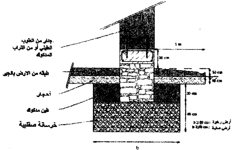
الشكل 49. أساس من خرسانة صقائية + ميطرات من الخرسانة المسلحة + أعمدة الربط جدار - ميطرة
