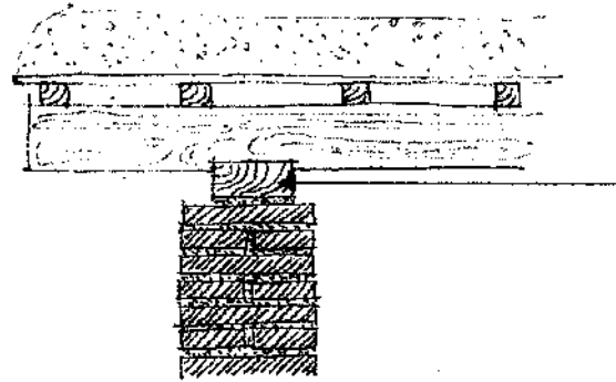
الشكل 18. ميطرة من خشب أو من خرسانة
