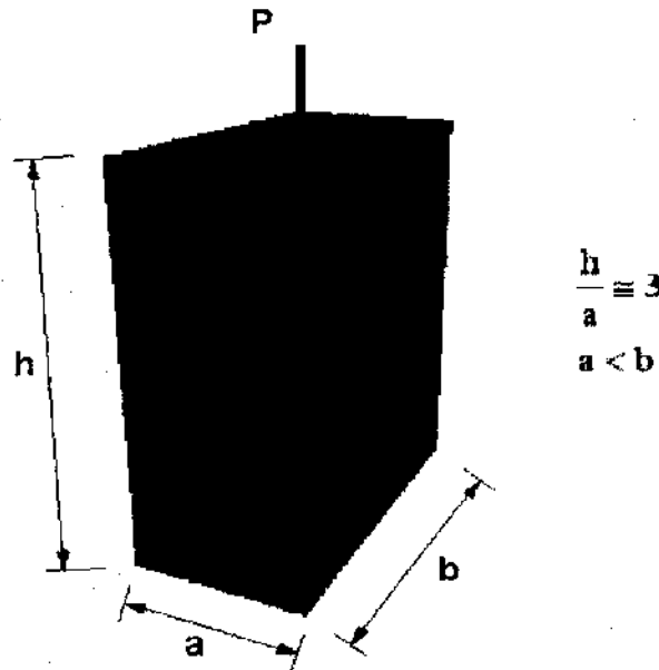
الشكل 15. حويطة لاختبار السحق عند الضغط
