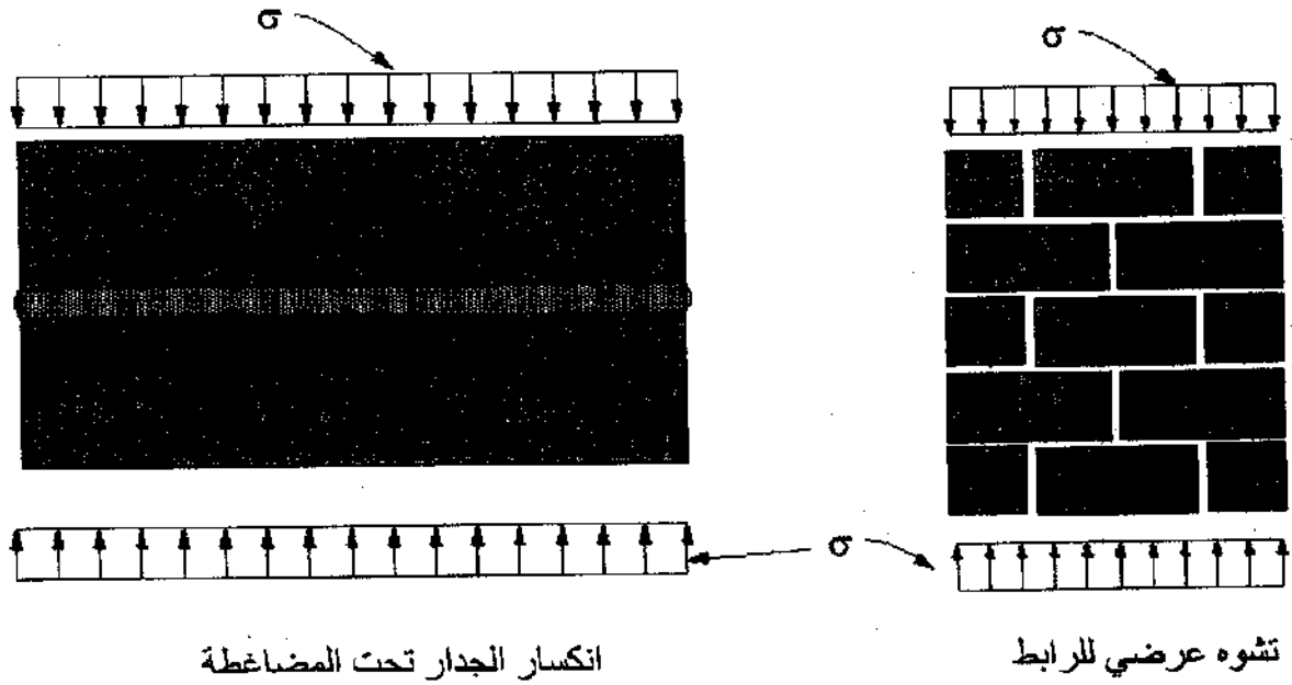
الشكل 22. انكسار البناء تحت مضاعطة بسيطة
