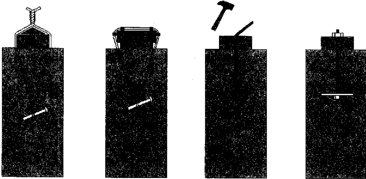
الشكل 41. أصناف الربط لميزرة أفقية لجدار
