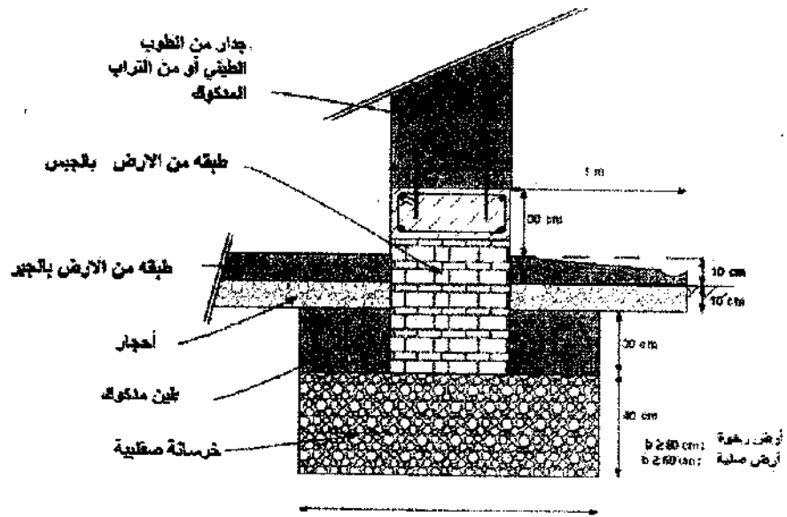
الشكل 50. أساس من خرسانة صقنوبية + ميترات من الخرسانة المسلحة + أعمدة الربط جدار - ميترية
