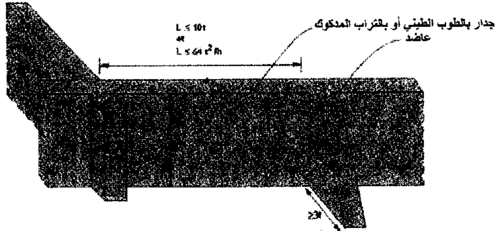
الشكل 32. الطول الأقصى لجدار بين العناصر الموطدة و/أو عارض من طين
